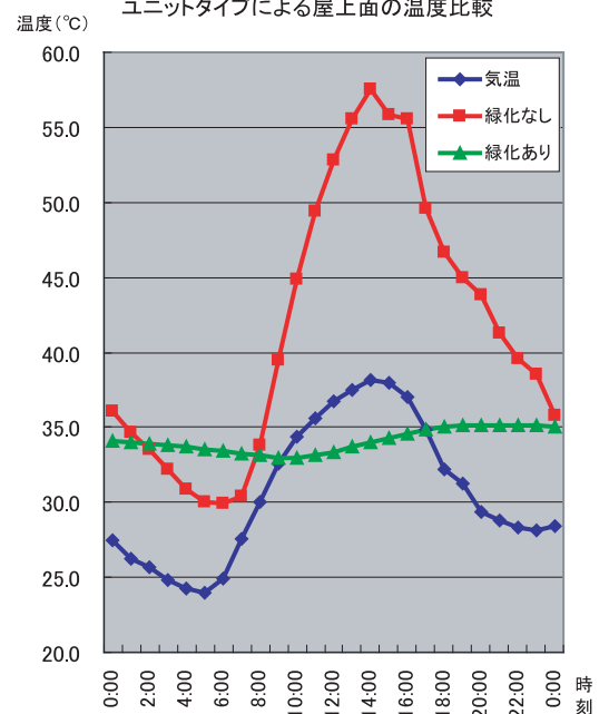
ユニットタイプによる屋上面の温度比較
