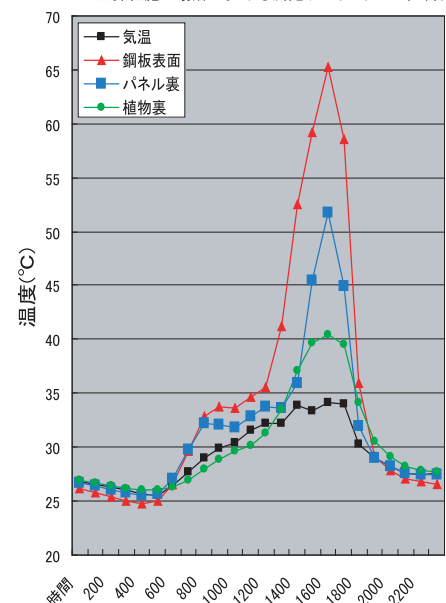
パネルタイプによる一日の壁面温度経時変化
